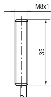
Габаритный чертеж
